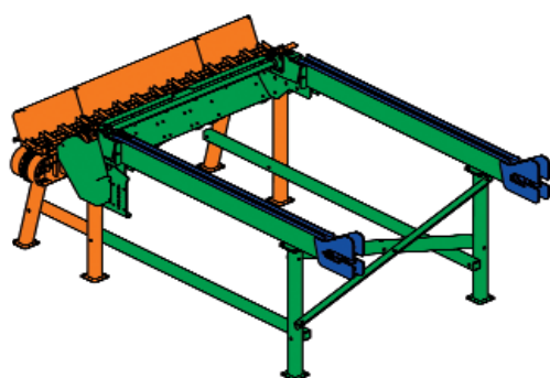
Uzdužni i poprečni transporter, stajaći model (za Spaltfix S-300, S-310 i S-320)
