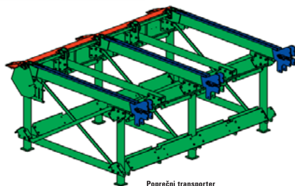
Poprečni transporter (za Spaltfix K-440 i K-450)
