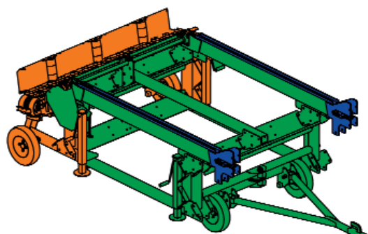
Uzdužni i poprečni transporter, sa šasijom (za Spaltfix S-300, S-310 i S-320)
