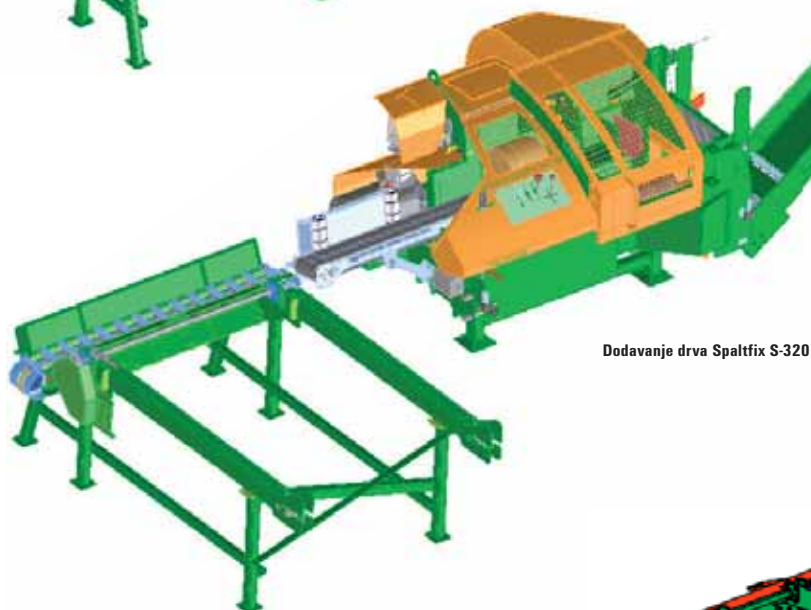
Dodavanje drva Spaltfix S- 300
